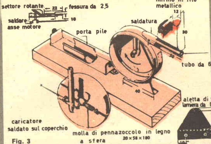
Fig. 3 - Vista del complesso lanciatore: il caricatore è aperto a mostrare l'interno.
