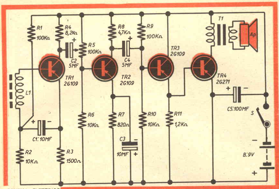
SCHEMA ELETTRICO
