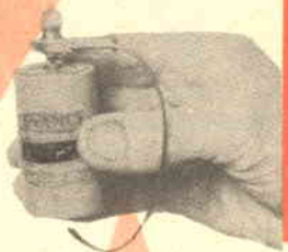
Fig. 1: Per provare rapidamente le pile, si può usare un filo d'acciaio, un coccodrillo ed una lampadina dell'adatta tensione; i tre, montati come si vede nella figura, costituiscono un tutto pratico e rapido nell'uso.
